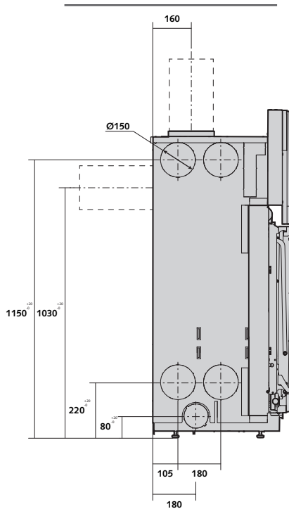
ZIJAAANZICHT
